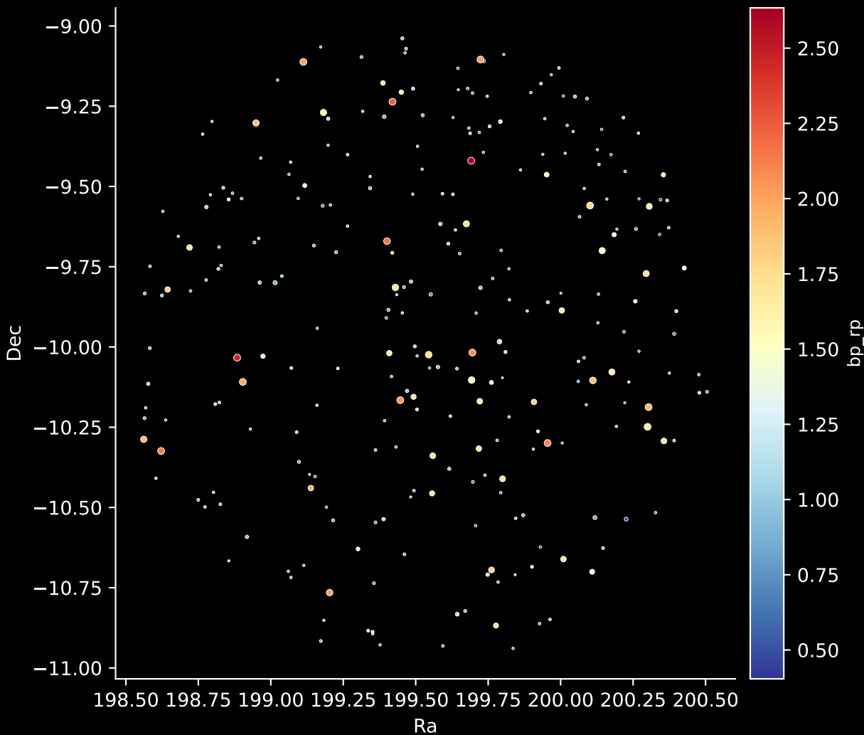
GALAH DR4 Field: [8893] Stars: 272
