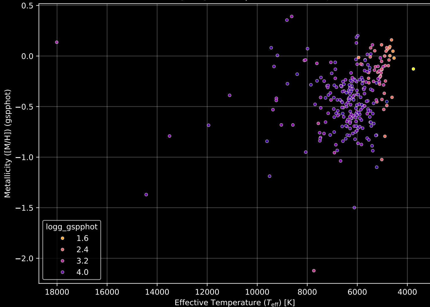
GALAH DR4 Field: [8893] Stellar Population Parameters (n= 272)
